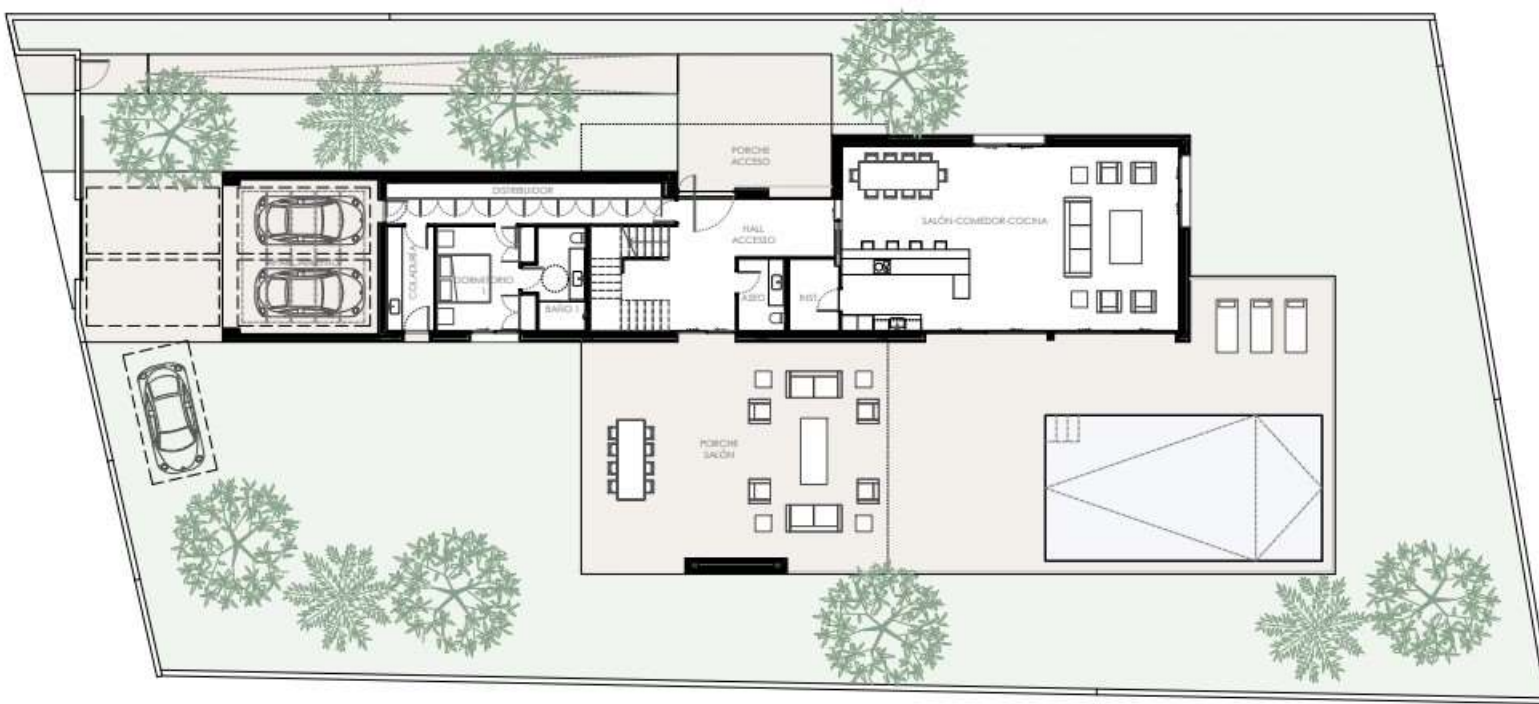
PLANTA BAJA
